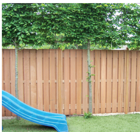
Hardhouten 21-planks met 3 tussen-regels en hardhouten palen 70 x 70 mm, 2.10 hoog
